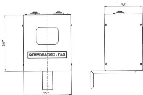
Рис. 1 – Габаритные размеры ящика
